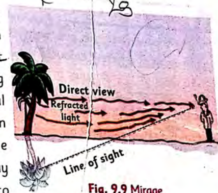
Fig. 9.9 Mirage
