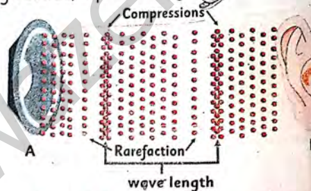
Fig. 10.1 Longitudinal sound wave
