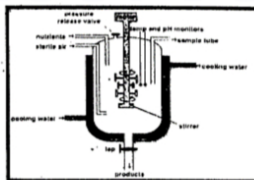
A batch fermenter
